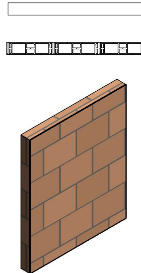
Bloque N° 4 de Perforación Vertical
